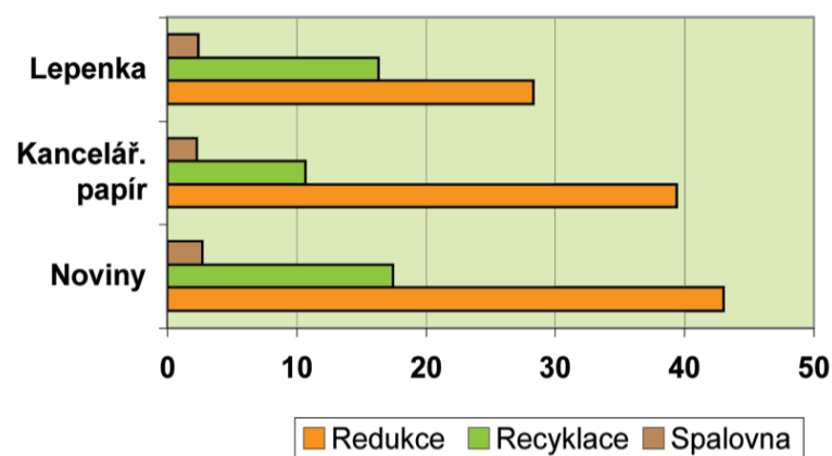
Úspory energie pro různé typy papíru [MJ/kg]
