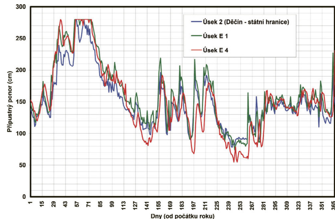
Přípustné ponory na kritických úsecích po výstavbě plavebního stupně Děčín (pozn.: hranice tzv. ekonomicky smysluplného ponoru, tedy ponoru, od kterého se již „vyplatí“ provozovat nákladní vodní dopravu, se udává 140 cm)
